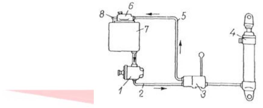
Emelőtargonca hidraulikus emelő-berendezésének vázlata 1. szivattyú; 2. nyomócső; 3. kapcsolószelep; 4. munkahenger; 5. visszafolyócső; 6. olajszűrő; 7. olajtartály; 8. légszűrő
