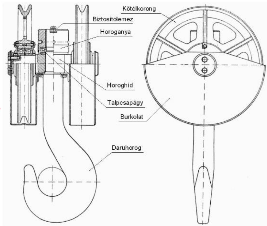
Horogszerkezet
