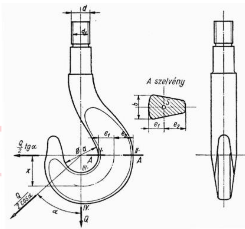
Egyágú horog
