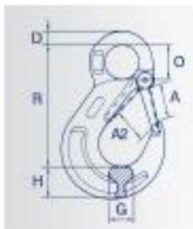
Kiakadástólóval ellátott biztonsági horog
