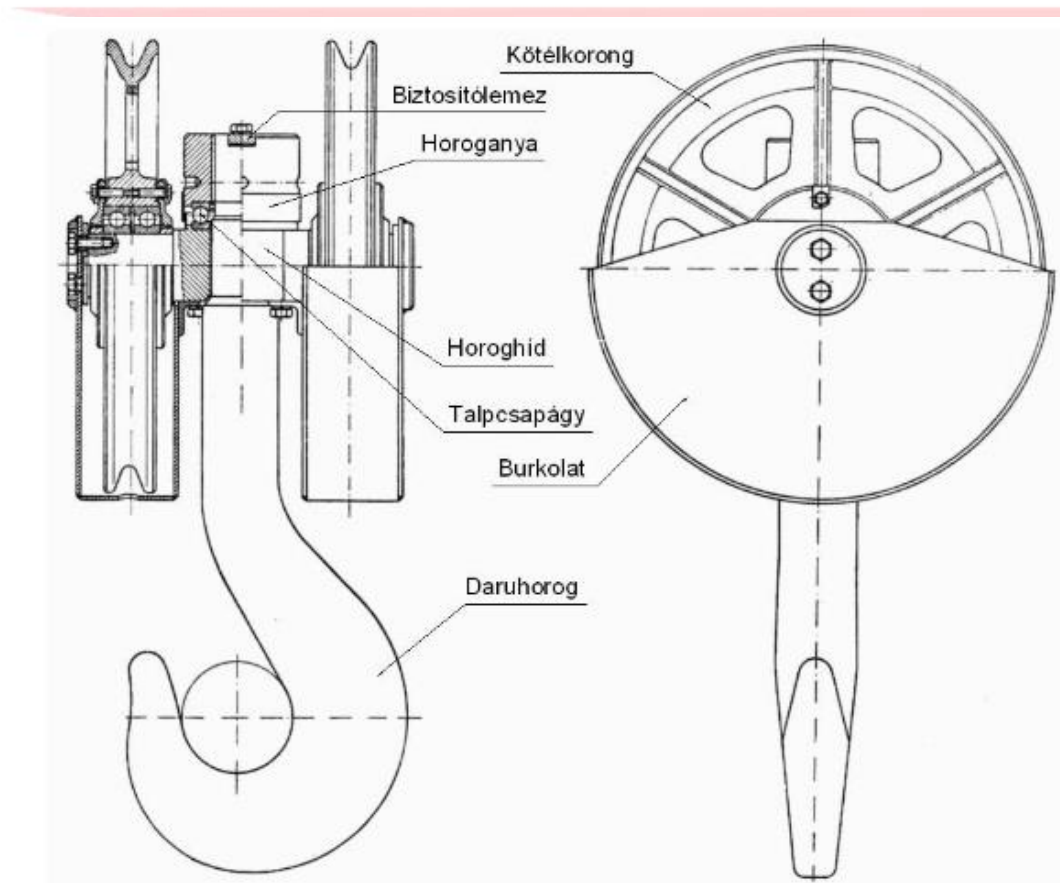
Horogszerkezet
