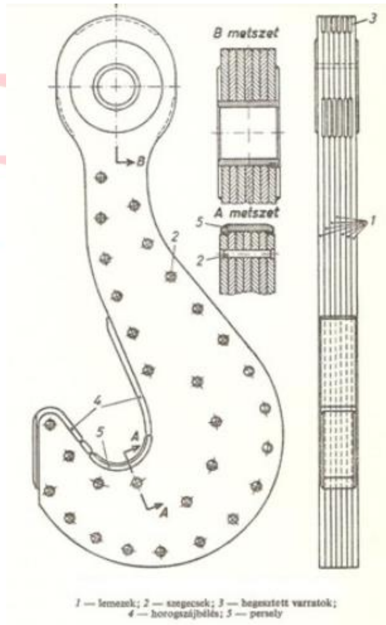
Lemezelt horog
