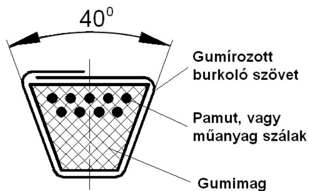
Az ékszíz kialakítása
