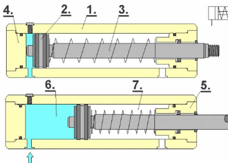
Egyszeres működésű munkahenger
