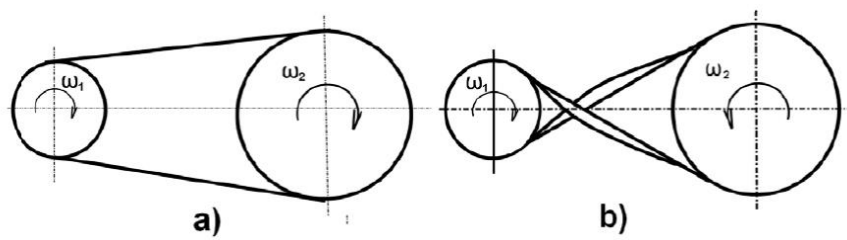
Nyitott (a) és keresztthajtás (b)
