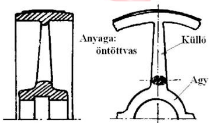
Szíjtárcsa
