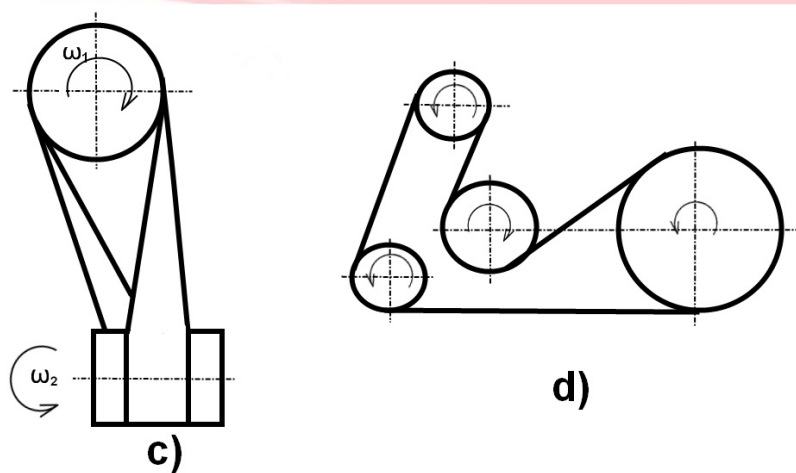
Kitérő tengelyű (c) és a terelősgörgős (d) hajtás
