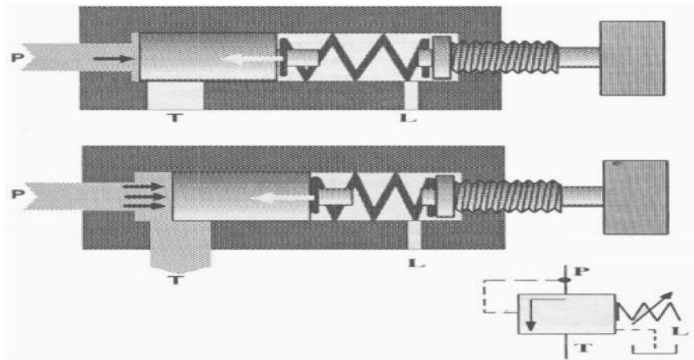
Nyomáshatároló szelep
